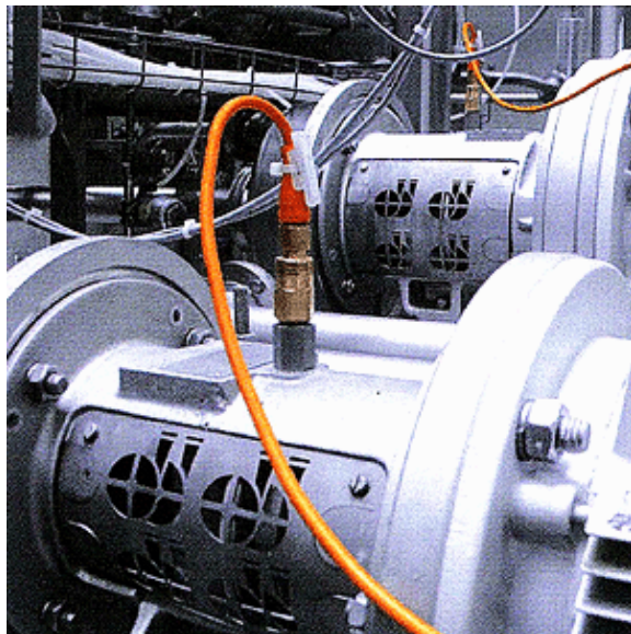
zapojenie snímača na meranom zariadení
